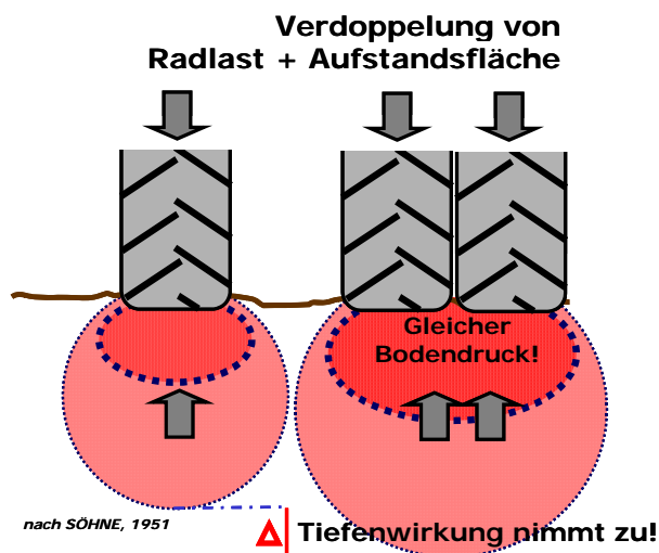
Abb. 4: Doppelte Radlast und verdoppelte Aufstandsfläche → größere Tiefenwirkung – trotz gleichen Kontaktflächendrucks!
