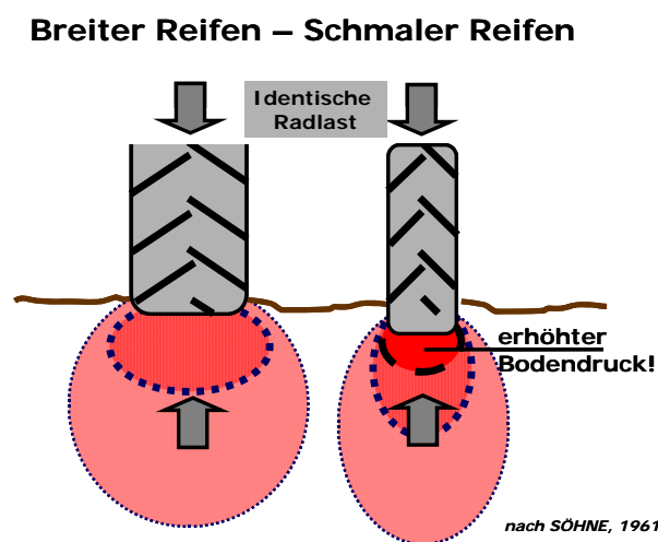
Abb. 2: Breiter Reifen → niedriger Bodendruck; schmaler Reifen → hoher Bodendruck!
